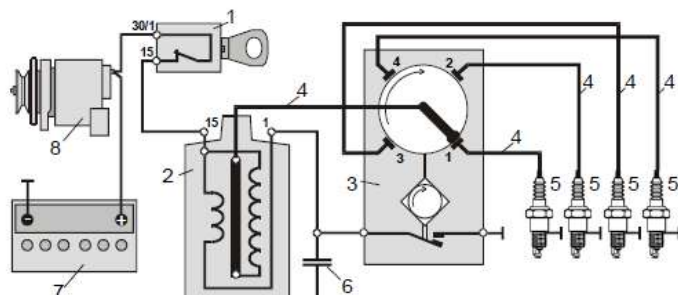
Рисунок 63. Схема контактной системы зажигания
