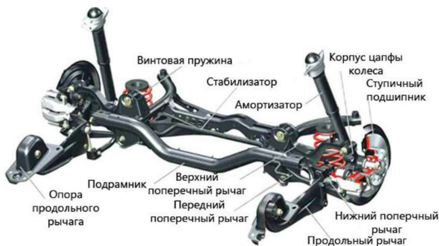
Рисунок 10. Многорычажная задняя подвеска
