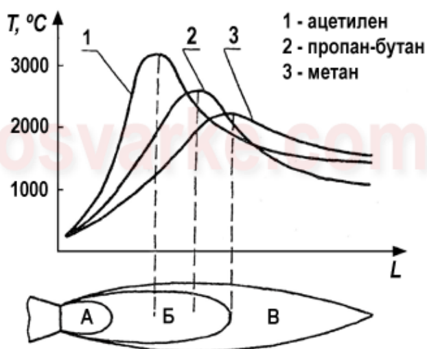
Рисунок 3 Строение газового пламени и распределение температур по его сечению
