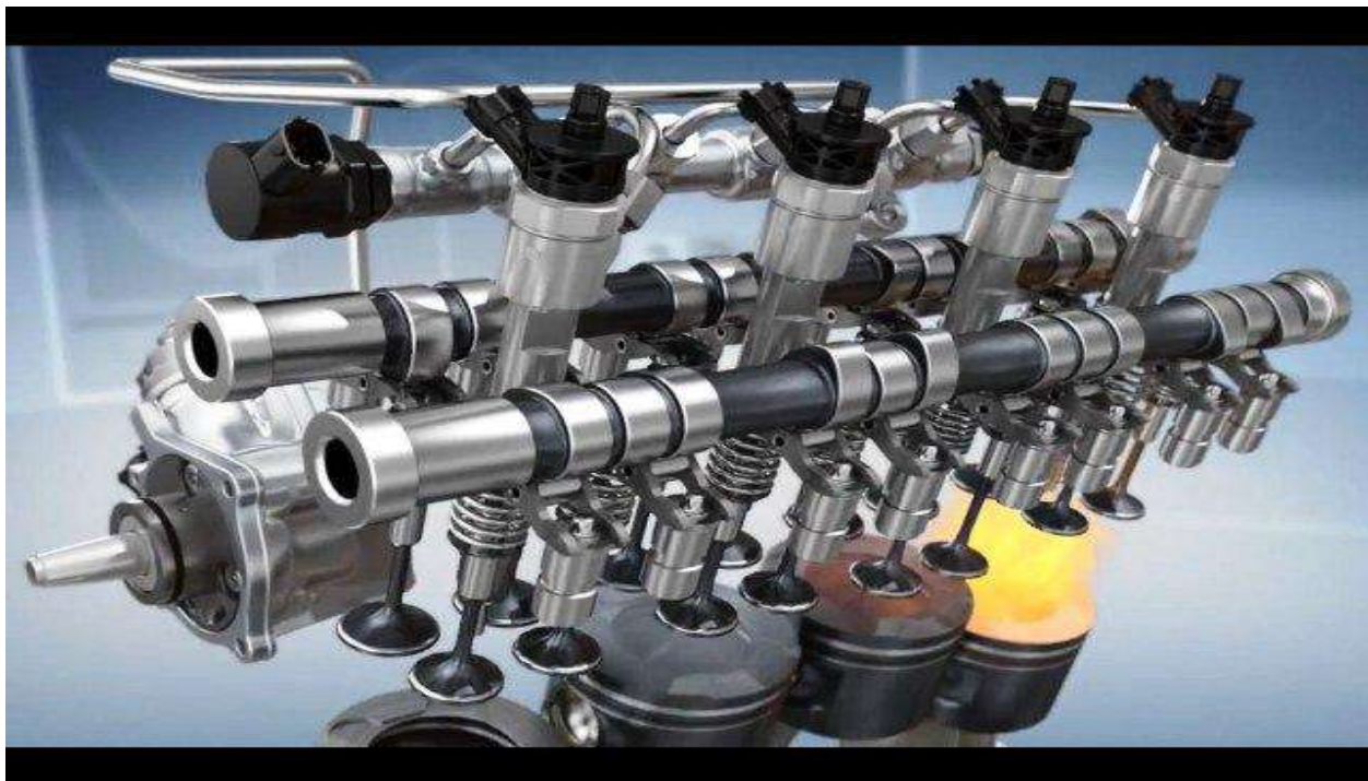
Рис.1 Газораспределительный механизм.
