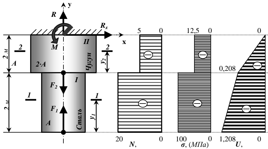
Рисунок– Построение эпюр продольных сил N , нормальных напряжений \sigma и перемещений U .
