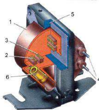
Рисунок 61 - Конструкция катушки зажигания 3112.3705
