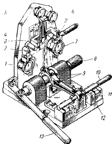
Рис. 13 Приспособление для контроля и правки шатуна:
