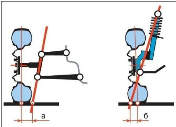
Рис. 15 Положительное (а) и отрицательное (б) плечо обката управляемого колеса
