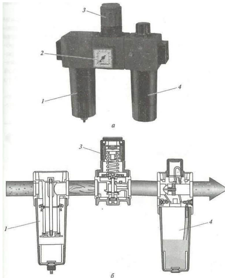
а — общий вид; б — конструкция в разрезе; 1- фильтр; 2 - манометр; 3 — регулятор давления; 4—лубликатор
