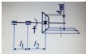
Рисунок 1 Схема входного вала
