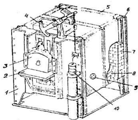
Рис. 4.2. Камерная печь.
