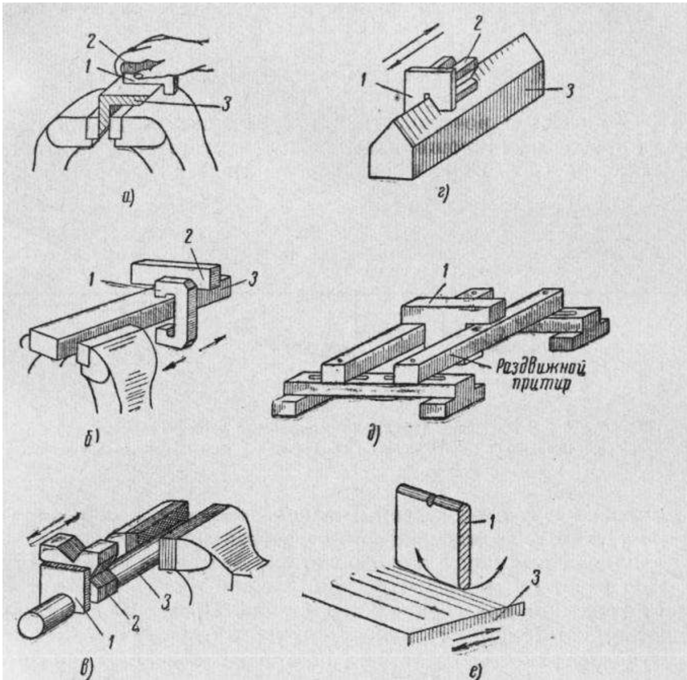
Рис. 3. Притирка внутренних мерительных поверхностей: а — шаблона (угольника), б — скобы, в — шаблона с полукруглой выемкой, г — углового шаблона (высотомера), е — шаблона с закруглениями; 1 — изделие, 2 — направляющий брусок, 3 — притир
