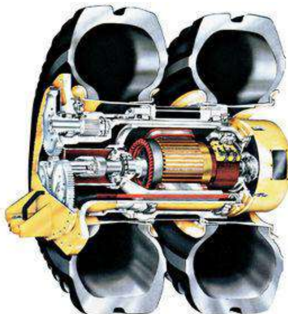
Рисунок 9 АКПП
