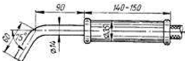
Рис. 12. Электрододержатель для безогарковой сварки
