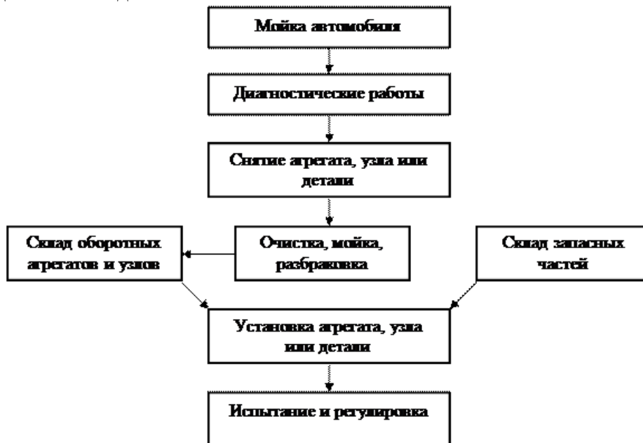
Рис. 1. Схема технологического процесса ремонта автомобилей в процессе их эксплуатации (постовые работы)
