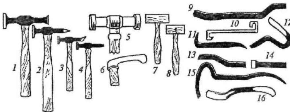
Рис. 4. Набор инструментов для удаления вмятин.
