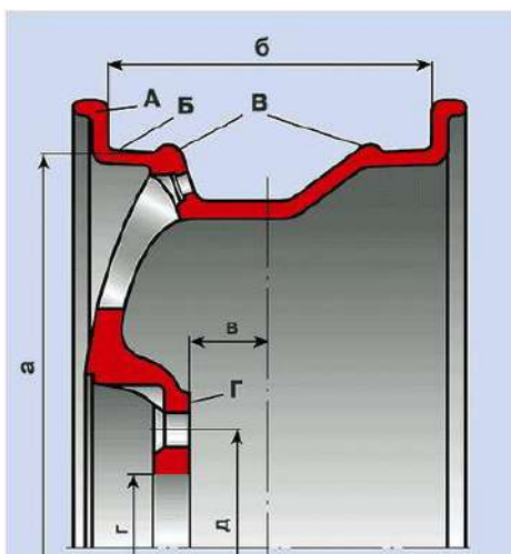
Рис 1. Основные элементы и размеры колеса легкового автомобиля: А – закраина обода; Б – полка; В – кольцевые выступы «хампы» для дополнительной фиксации бортов бескамерной шины; Г – плоскость крепления; а – монтажный диаметр; б – ширина обода; в – вылет (ET – расстояние между плоскостью симметрии обода и крепежной плоскостью колеса); г – диаметр центрального отверстия под ступицу (DIA); д – диаметр окружности расположения центров крепежных болтов или шпилек (PCD)
