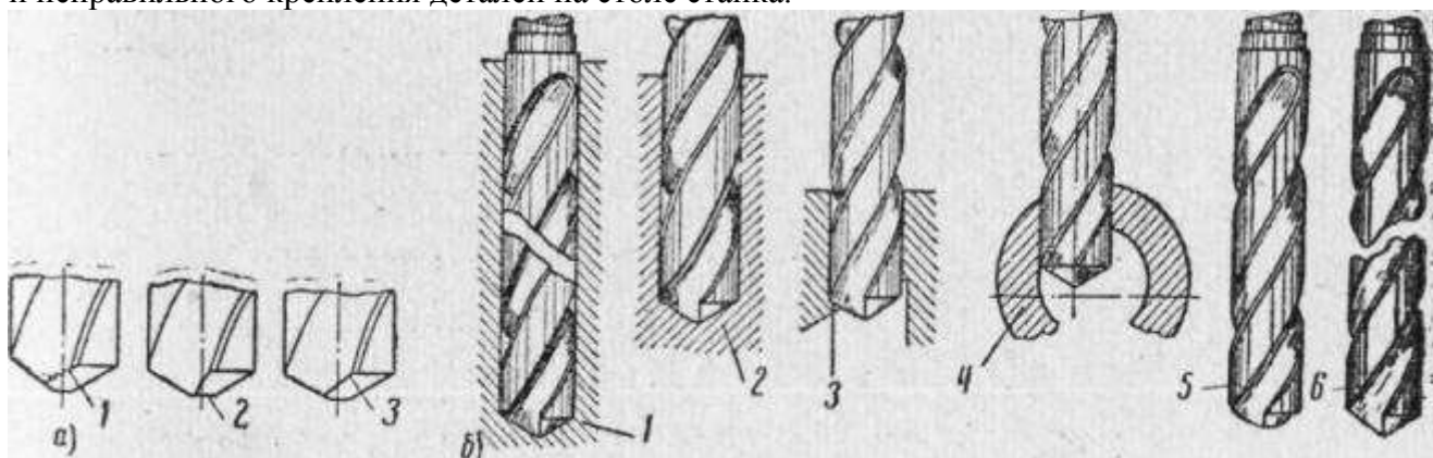
Рис. 2. Затупление и поломка сверл: а —участки, подвергающиеся затуплению: 1 — выкрошенная режущая кромка, 2 — затупленная поперечная кромка, 3 — затупленный угол; б —примеры поломки сверл: 1 — сверло глубоко вошло в отверстие, не выходит стружка, 2 — сверло натолкнулось на постороннее твердое включение, 3 — неравномерный выход сверла из отверстия по его окружности, 4 — нецентральный выход сверла из отверстия, 5 — затупление сверла под влиянием чрезмерно большой скорости резания, 6 — поломка сверла вследствие чрезмерно большой подачи
