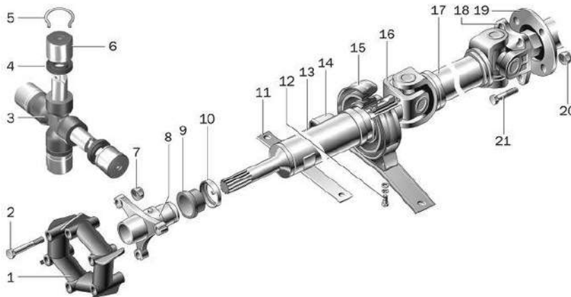
Рис. 2 Карданная передача:
