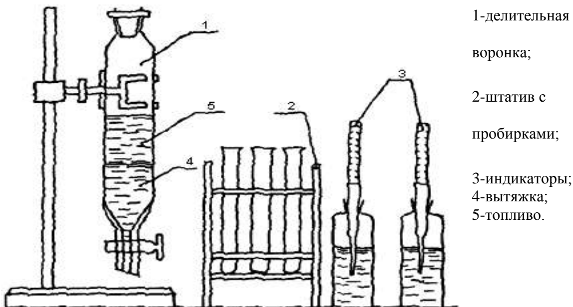
Рис.1 Прибор для определения в топливе ВКЩ.
