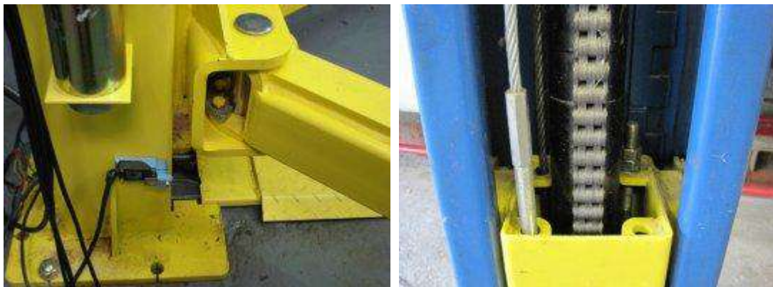
Рисунок 11. Привод подъемников
