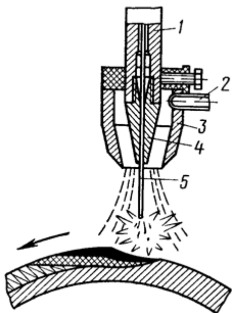
Рис. 20.3. Схема установки для наплавки в среде защитных газов: 1 – мундштук; 2 – сопло для подачи защитного газа; 3 – газовое сопло; 4 – наконечник; 5 – электродная проволока;
