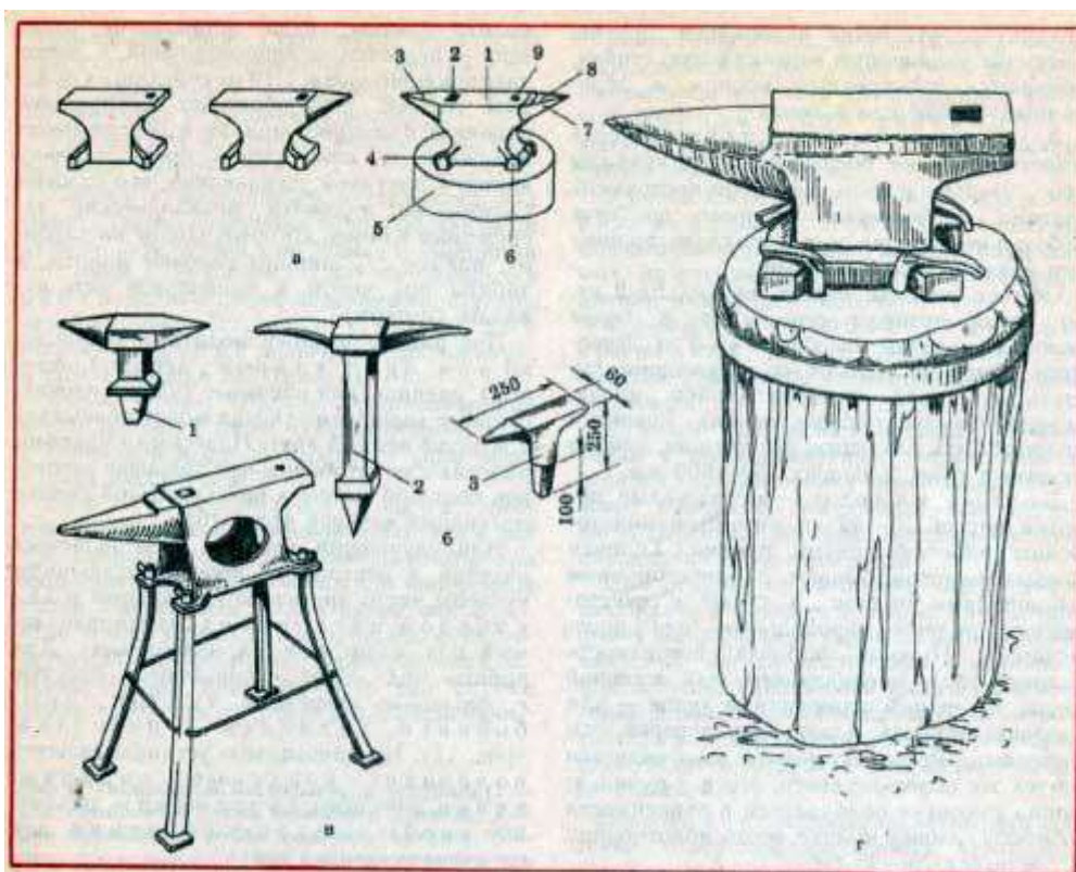
Рис.3. Наковальни и шпераки: а — безрогая, однорогая и двурогая наковальни (1 — лицо; 2 — квадратное отверстие; 3 — хвост; 4 — скобы; 5 — стул; 6 — лапы; 7 — конический рог; 8 — незакаленная площадка; 9 — круглое отверстие); б — шпераки (1 — вставляемый в наковальню; 2 — вбиваемый в землю; 3 — для мелких работ); в — переносная наковальня; г — наковальня, укрепленная на стуле
