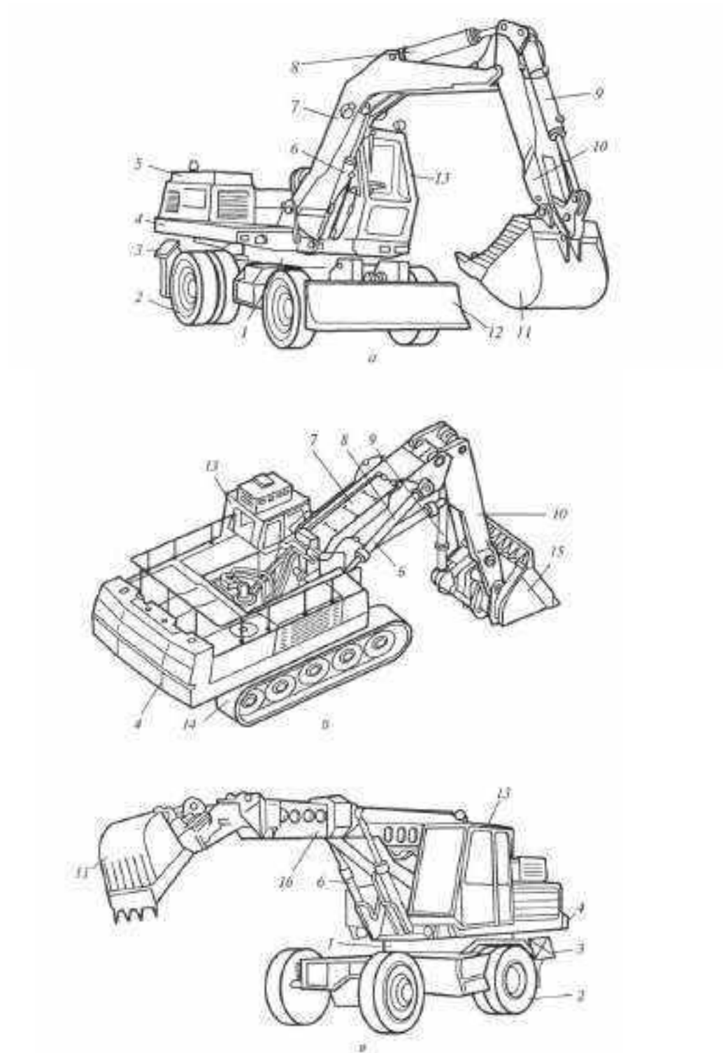
Рисунок 7. - Одноковшовые гидравлические полноповоротные экскаваторы с жесткой подвеской рабочего оборудования:
