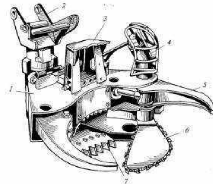
Рис. 3.8. Захватно-срезающее валочное устройство машины ЛП-17: 1 — корпус; 2 — подвеска; 3 — сварная призма; 4 — гидромотор привода пилы; 5 — захват; 6 — пила; 7 — гидродомкрат
