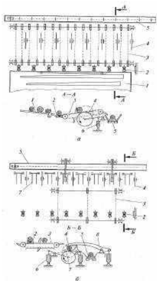
Рис. 3. Раскряжечные установки с поперечным перемещением хлыста:
