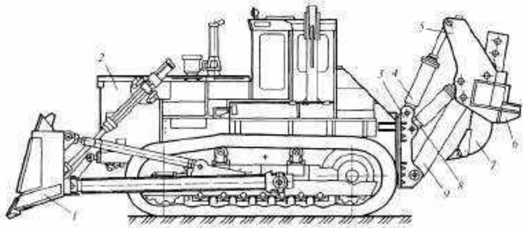
Рис. 4.13. Бульдозер-рыхлитель на базе трактора Т-35.01 1 — бульдозерное оборудование (полусферический отвал), 2 — трактор, 3 — опорный кронштейн, 4 — гидромеханизм регулирования угла рыхления, 5 — рабочая балка, 6 — буферное устройство, 7 — зуб, 8 — гидродвигатель балки — опускания рыхлителя, 9 — шнековая лопата
