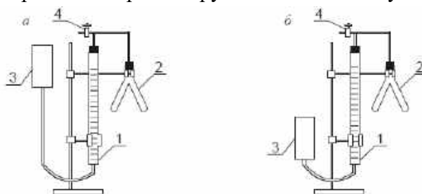
Прибор для определения активности катализатора:
