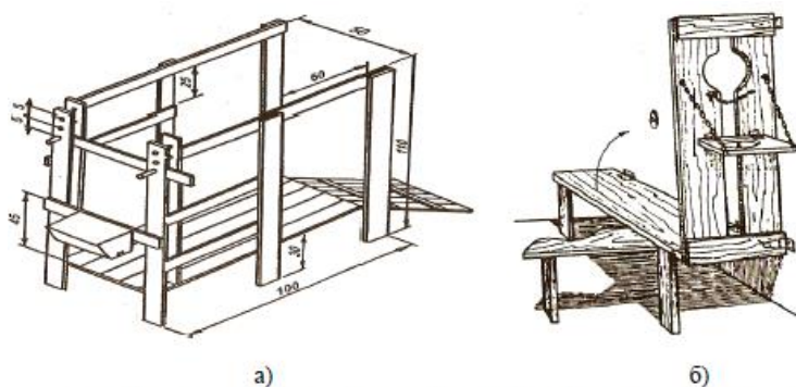
Рисунок 46 – Дойльные станки: а) с приподнятым полом; б) складной
