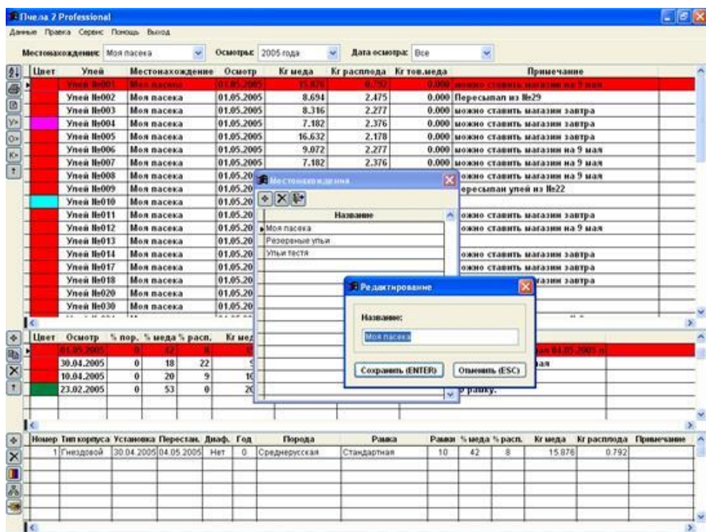
Рисунок 6 – Справочник «Местонахождение».
