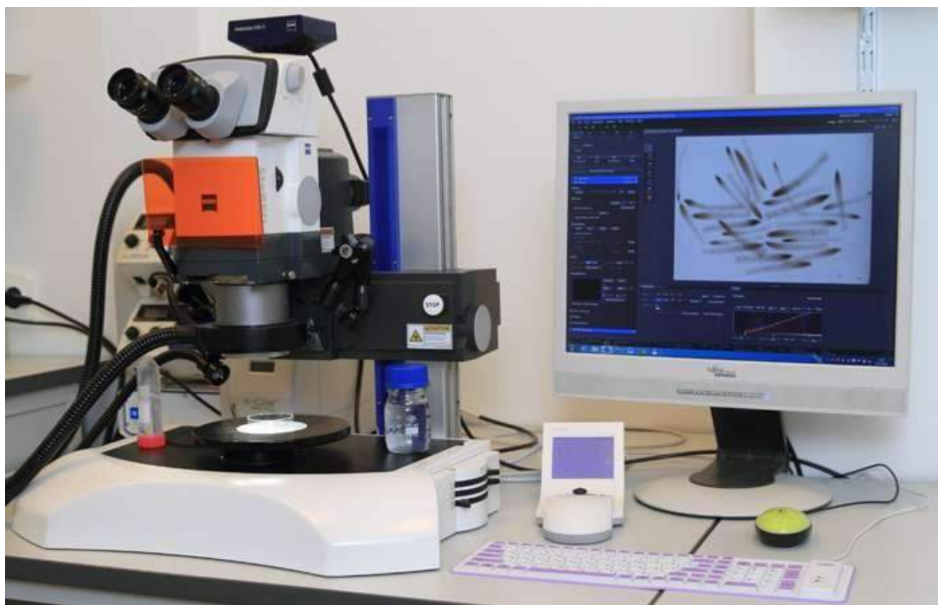
Рисунок 34 - Люминесцентный микроскоп.
