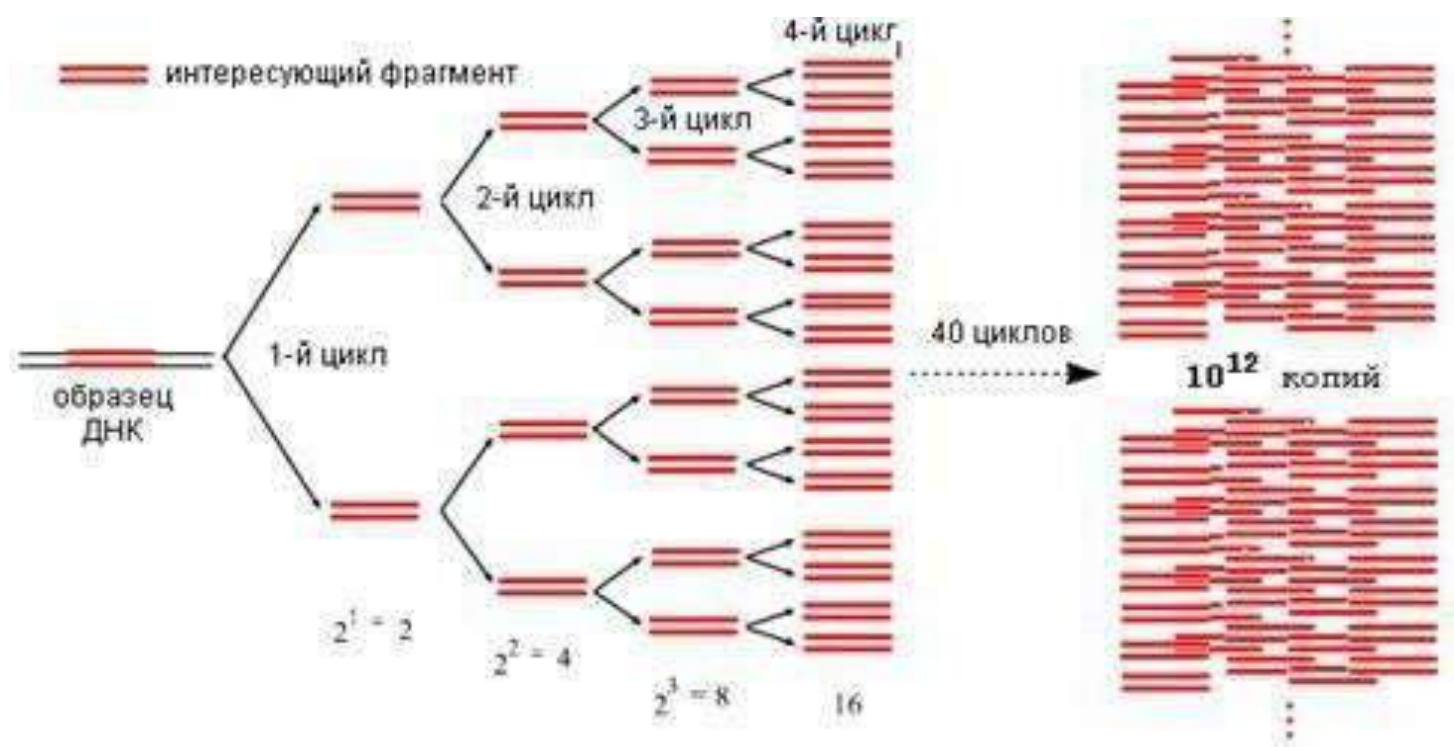
Рисунок 42 - Циклы ПЦР.
