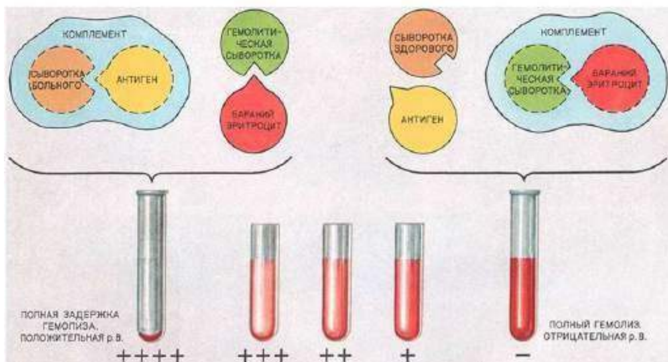
Рисунок 76 - РСК (принцип).
